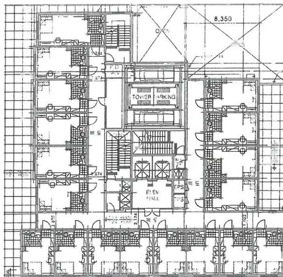
[제3~11층 내부구조도]
